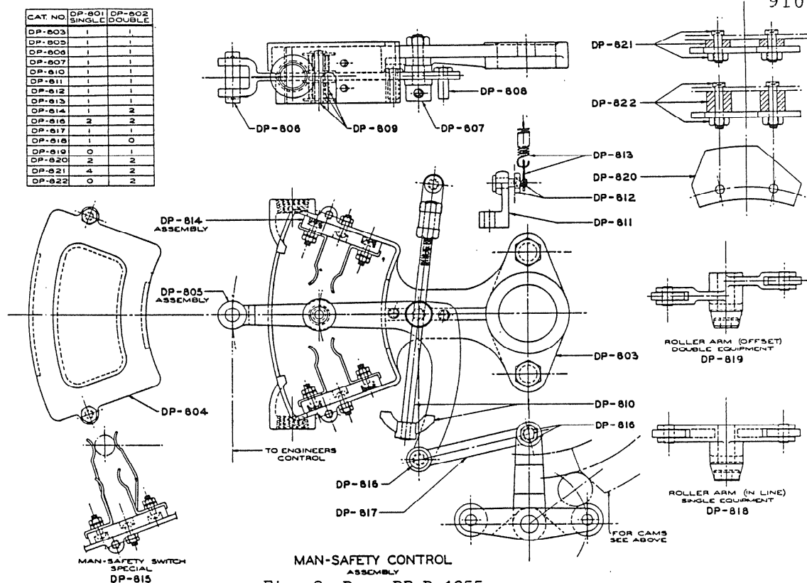
Fig. 8 Drg. DP-D-1255
