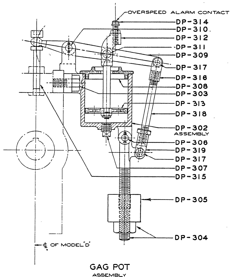
Fig. 3 Drg. DP-D-1252
