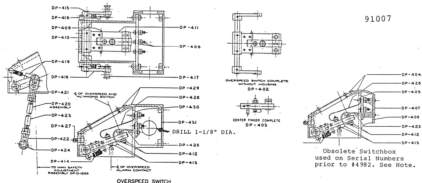
Fig. 4 Drg. DP-D-2207
