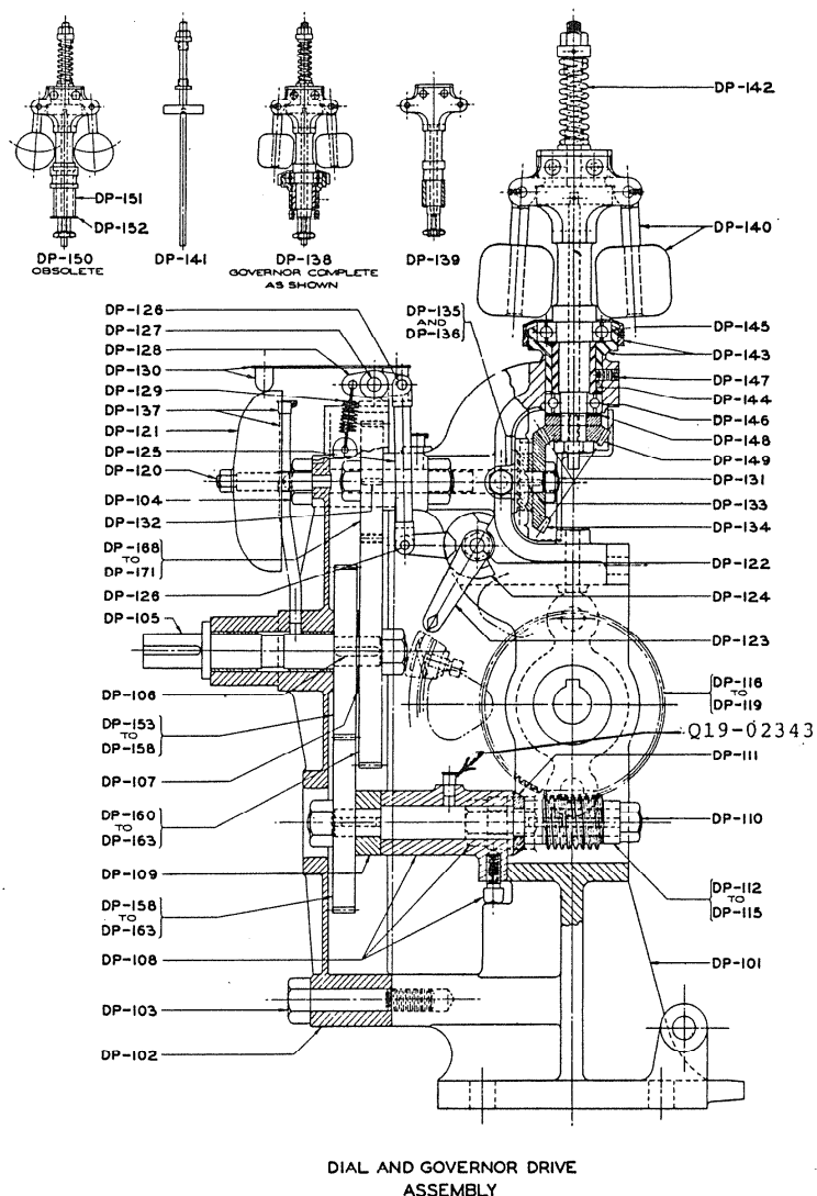
Fig. 1 Drg. DP-D-2153
