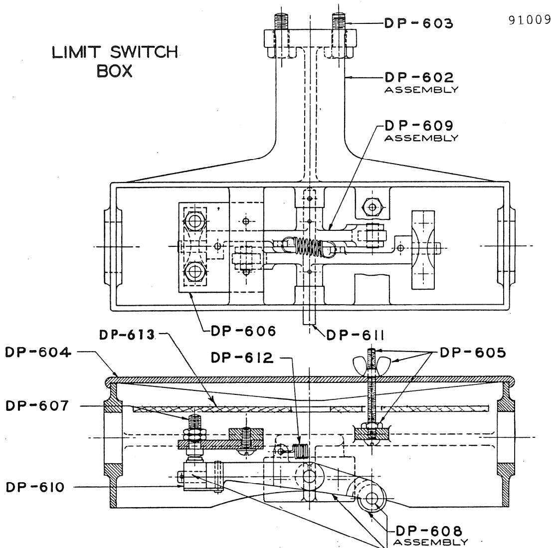
Fig. 6 Drg. DP-D-1254
