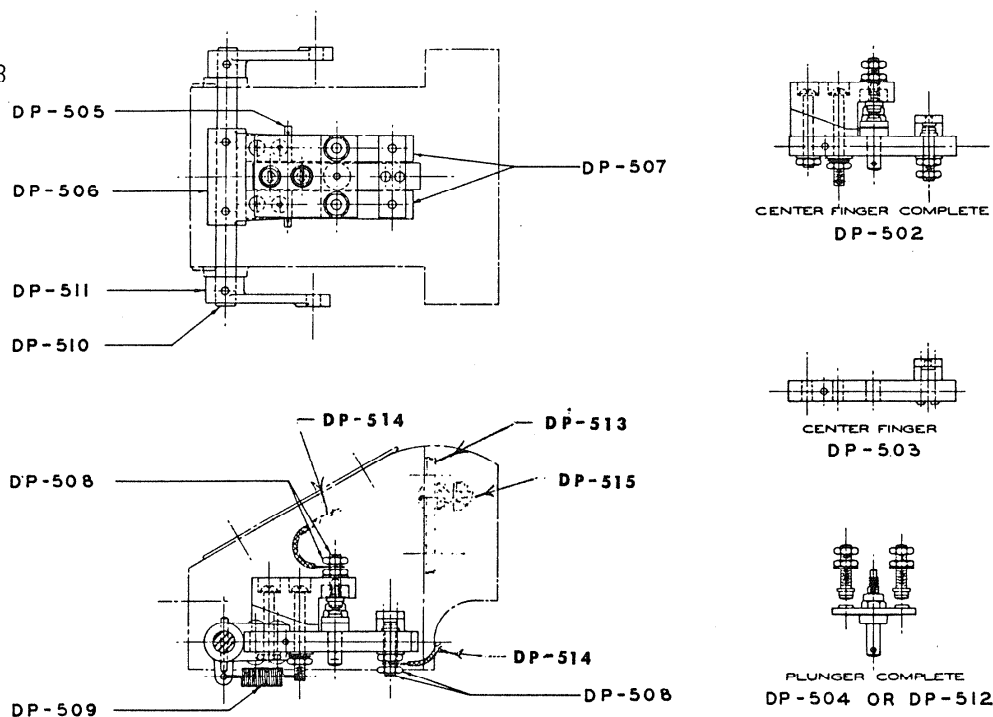
Fig. 5 Drg. DP-D-1960
