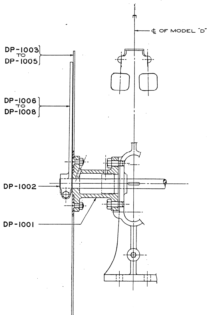
Fig. 10 Drg. DP-D-1230
